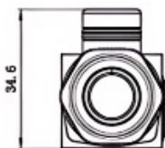
插头除键槽及类型标识不同外，其它结构均相同
